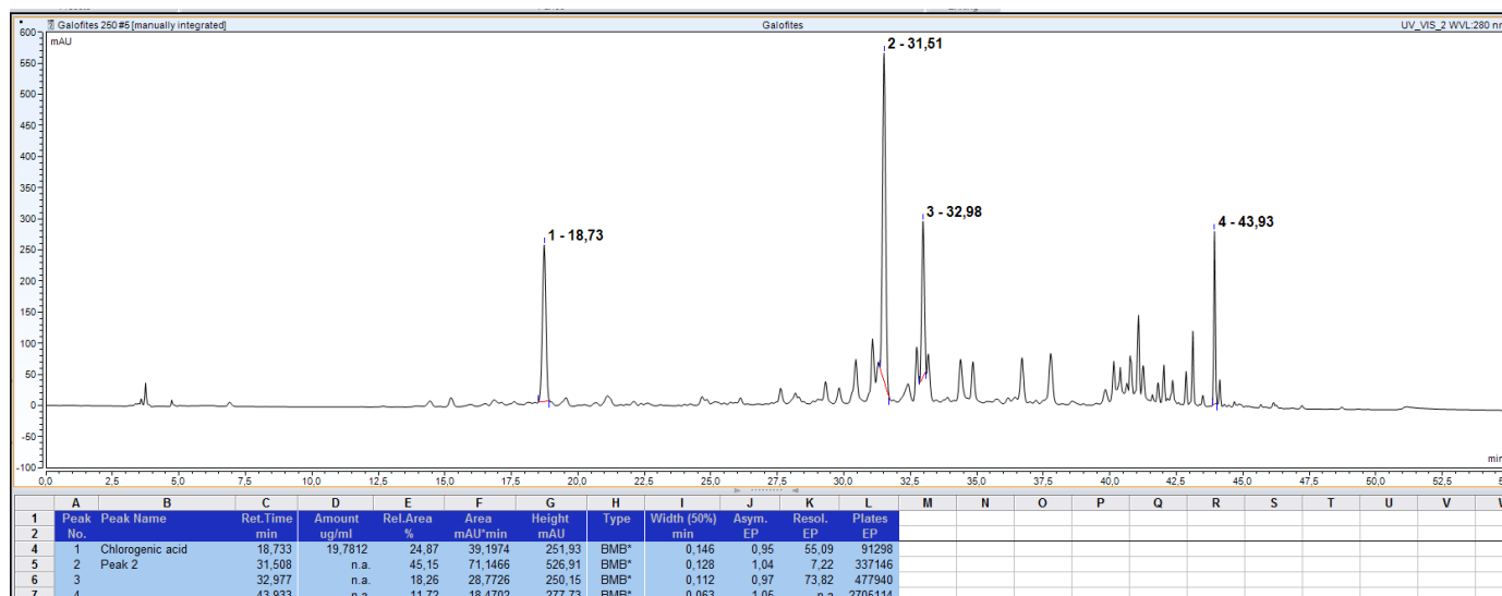
Рис. 2. — Хроматограмма надземной части полыни Artemisia santonica L. после хранения растения в течение 10 дней (280 нм).
