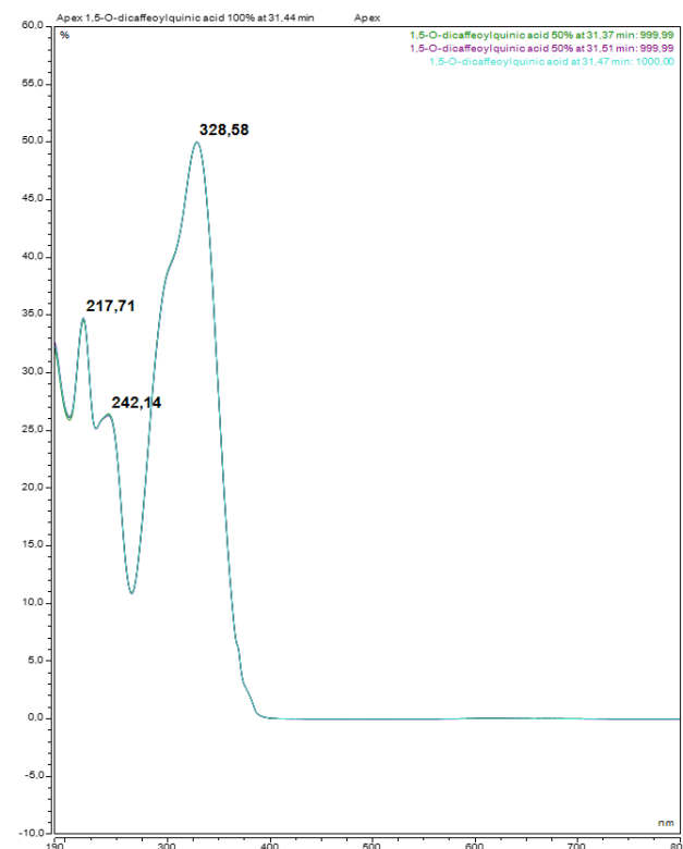
Рис. 4. — Спектр 1,5-ди-О-кофеилхинной кислоты в диапазоне 190–800 нм.
